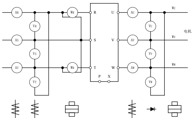
图 10-7 主电路功率测定电路
